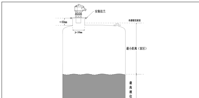
直接将仪表安装在平顶容器上
