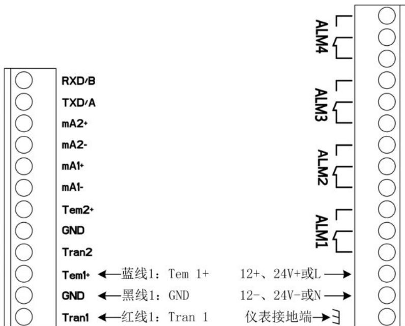
分体式超声波物位计接线图
